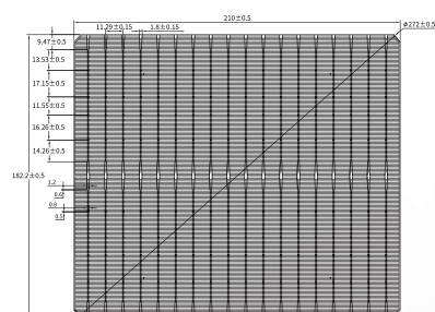
電池背面 Rear side
