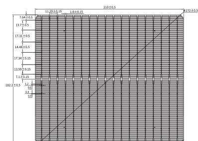
電池正面 Front side
