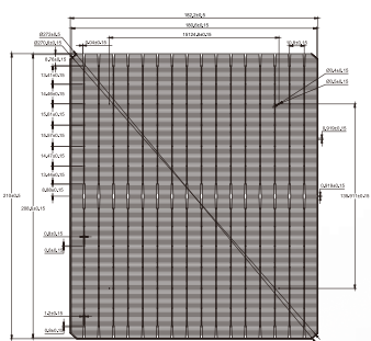
電池背面 Rear side
