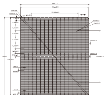
電池正面 Front side
