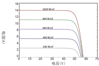
不同辐照度下 电流-电压曲线图
