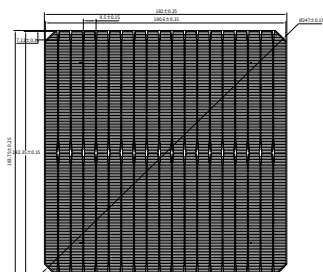
電池正面 Front side
