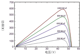
不同辐照度下 功率-电压曲线图
