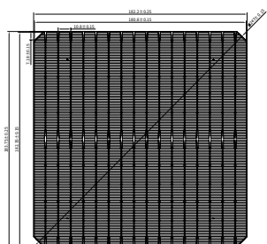
電池正面 Front side
