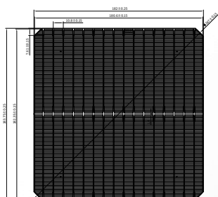
電池背面 Rear side
