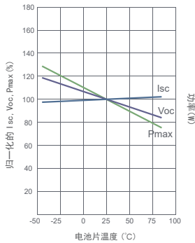
不同温度下的Isc、Voc、 Pmax的温度曲线图
